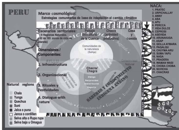
Figura 2. Marco cosmológico
